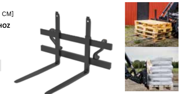
Kapható kiegészítők: Rönkfogó / hidraulikus megfogó (1.) Bálatúske (2.) Adapter hidraulikus villakar állításhoz (3.) Villakar hosszabbítás (2 m) (4.)
